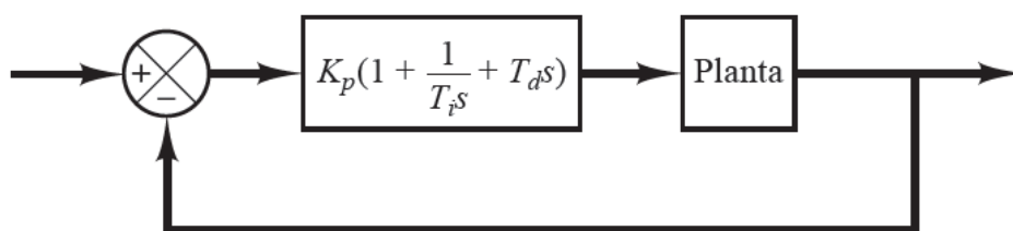
Figura 3 – Diagrama de blocos de um sistema malha fechada com controlador PID (OGATA, 2010).
