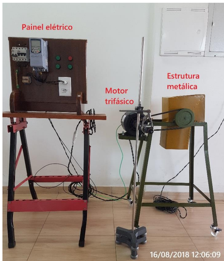
Figura 16 – Protótipo do painel elétrico e do ralador de mandioca.
